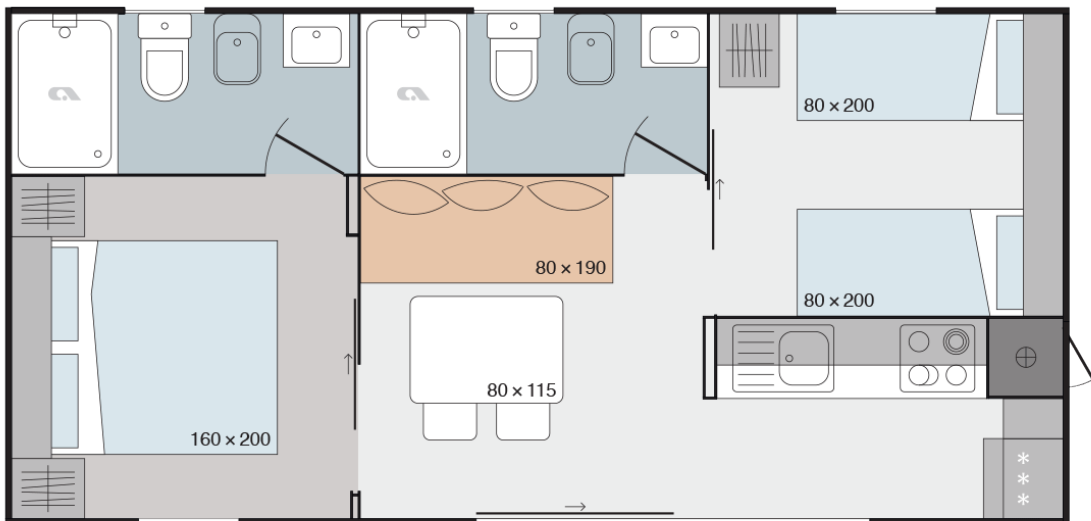
MLine 804 F22
